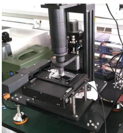
全自动荧光成像系统
